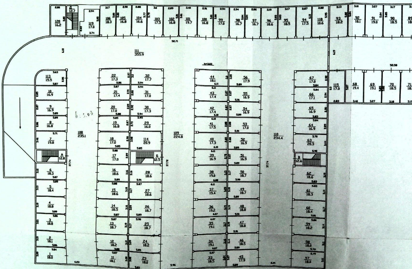
ПОЭТАЖНЫЙ ПЛАН СТРОЕНИЯ ЛИТ. Б находящегося в г. Мытицы, проезд 3825
